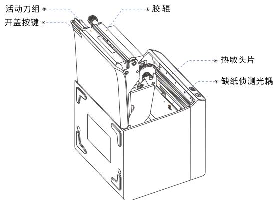
内视图
