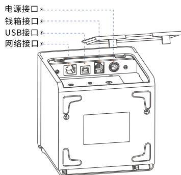
后视图
